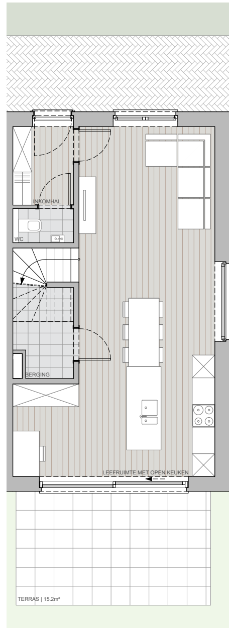
GRONDPLAN Niv. 0
